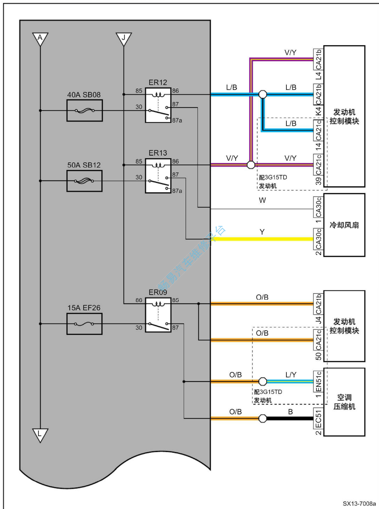
前机舱保险丝、继电器盒电源分布图 (续7)
