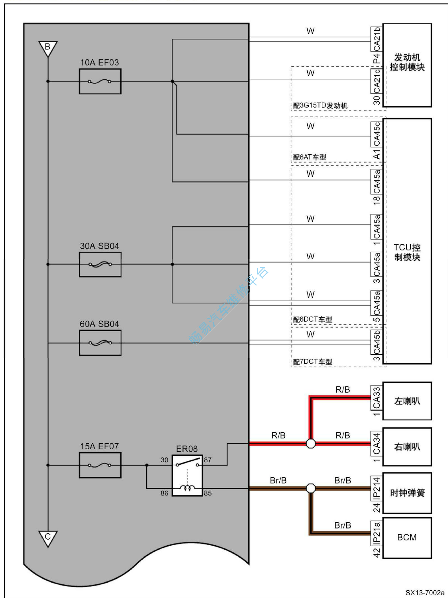
机舱保险丝、继电器盒电源分布图 (续1)
