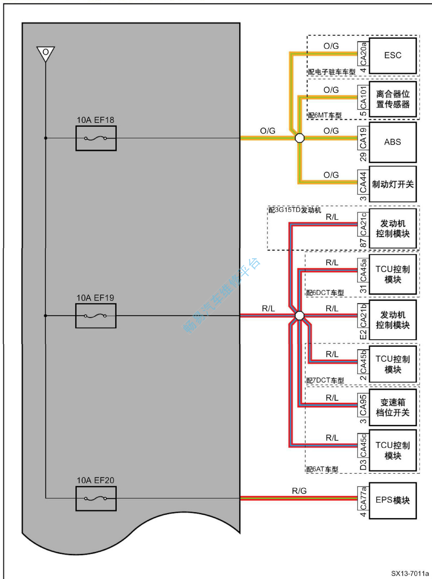
前机舱保险丝、继电器盒电源分布图 (续10)
