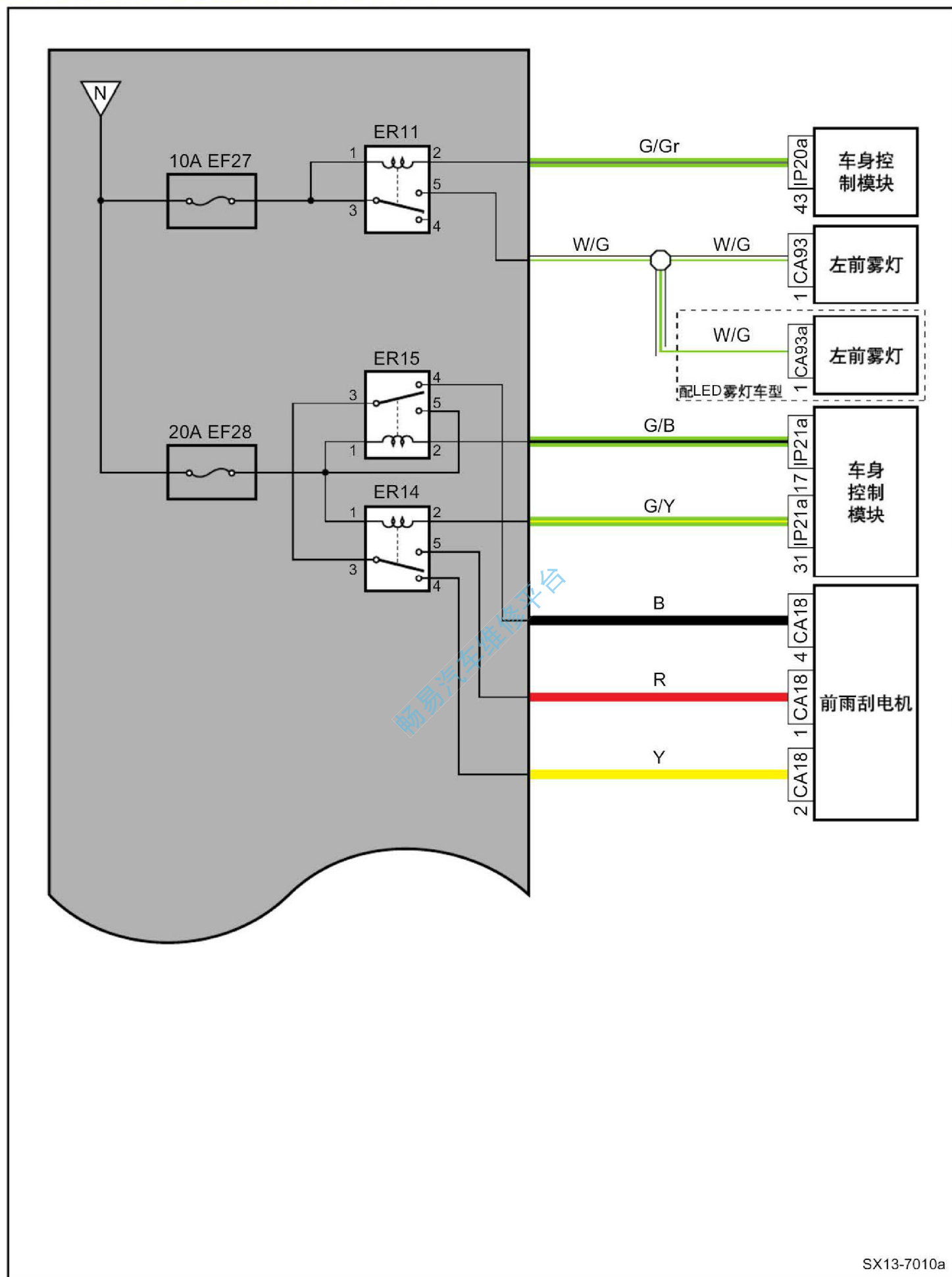
前机舱保险丝、继电器盒电源分布图 (续9)
