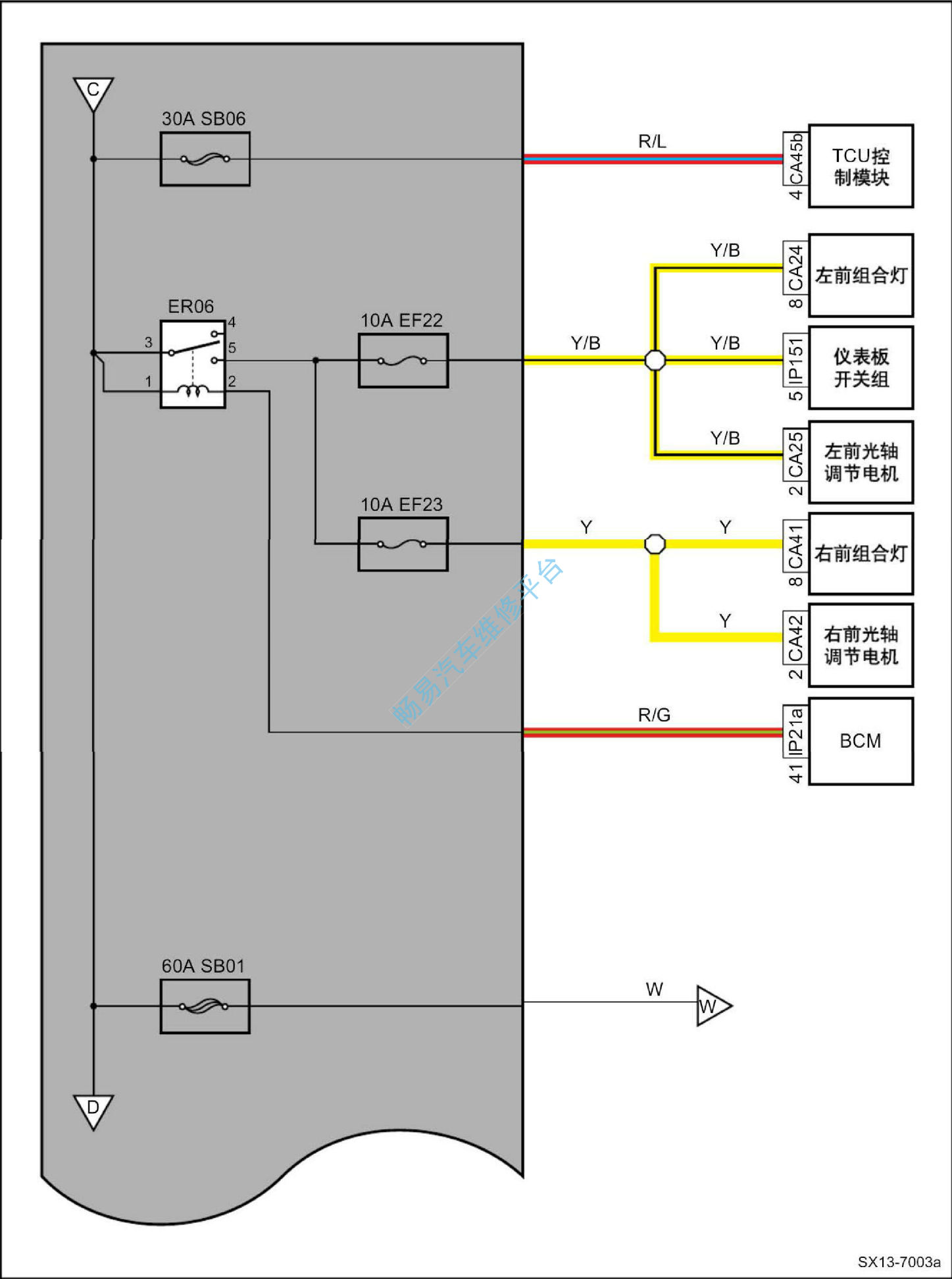
前机舱保险丝、继电器盒电源分布图 ( 续2 )
