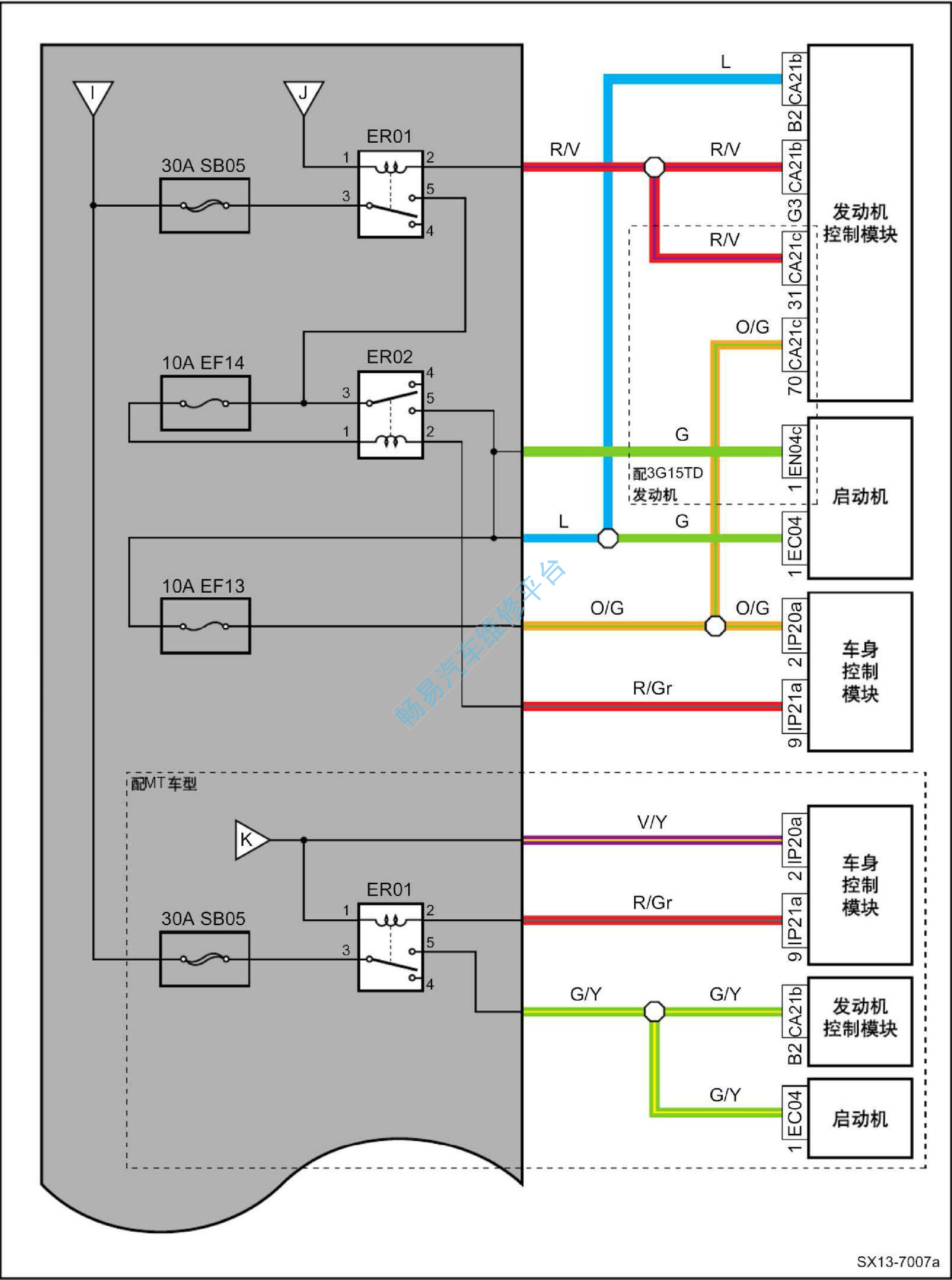
前机舱保险丝、继电器盒电源分布图（续6）
