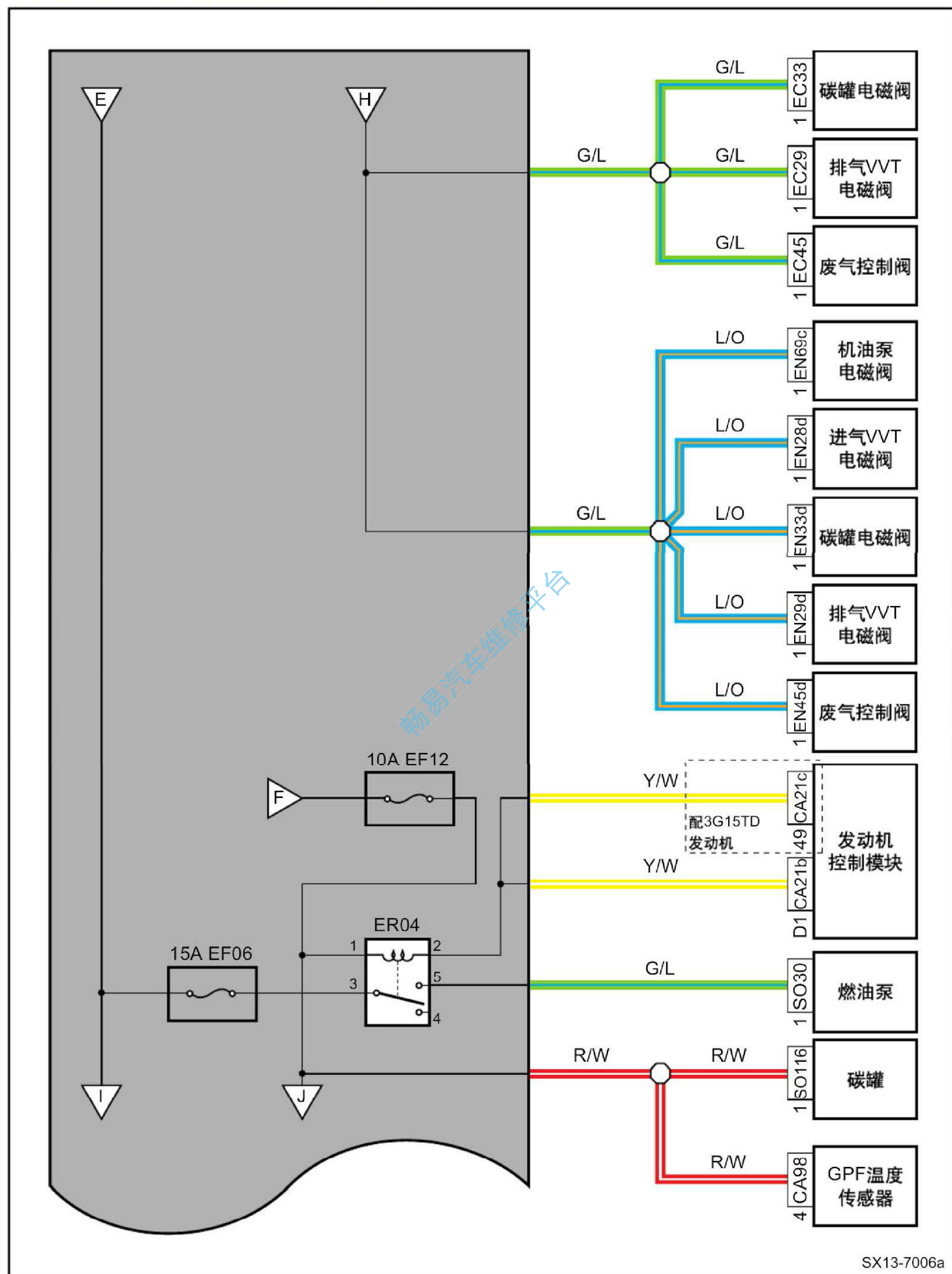
前机舱保险丝、继电器盒电源分布图 (续5)
