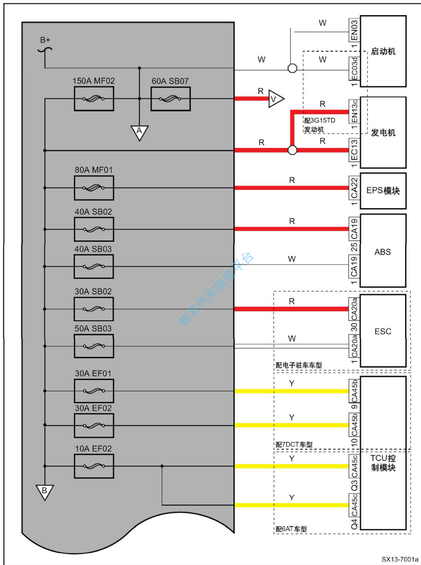
前机舱保险丝、继电器盒电源分布图
