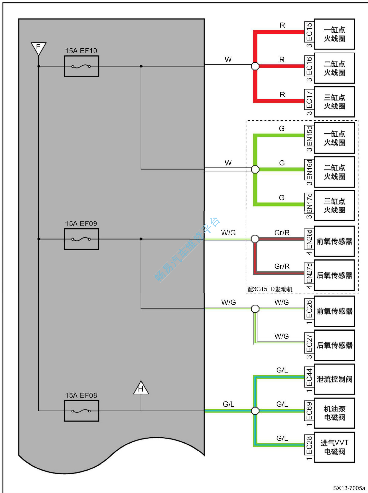
前机舱保险丝、继电器盒电源分布图 (续4)
